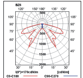
Für die Gänge: RETTO AB 1x3W, LED
