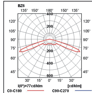
Für offene Flächen: RETTO AB 1x3W, LED
