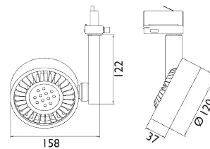
Tikon M Maße:
