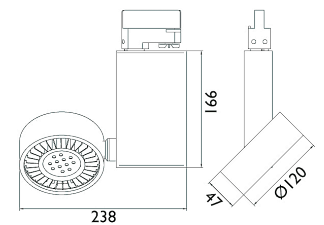
Tikon L Maße:
