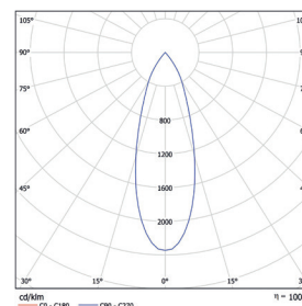
TRITON 3 Anbau 40°, 35W/830
