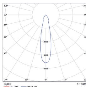
TRITON 3 Anbau 24°, 35W/830
